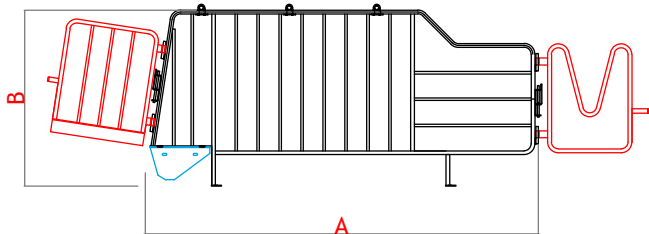
Модель STANDARD EVOTECK из арматурного прутка
